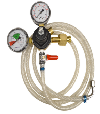
REGULADOR DE PRESION CO2 CON ACCESORIOS
