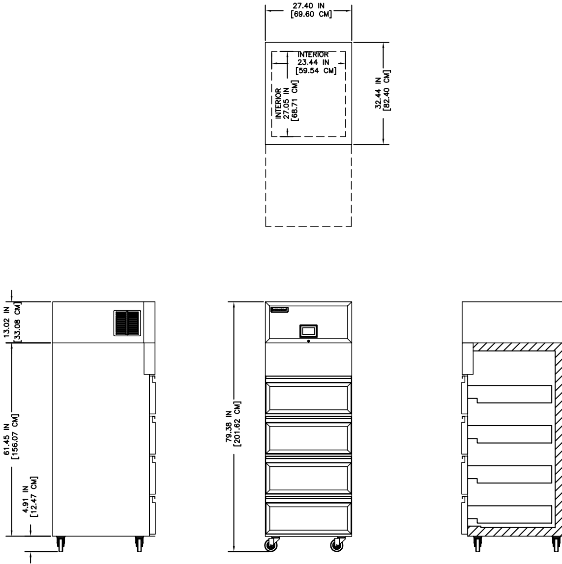
TYP. LEFT END VIEW
