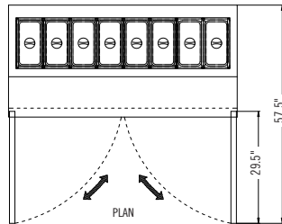
VALSL-2D-60
